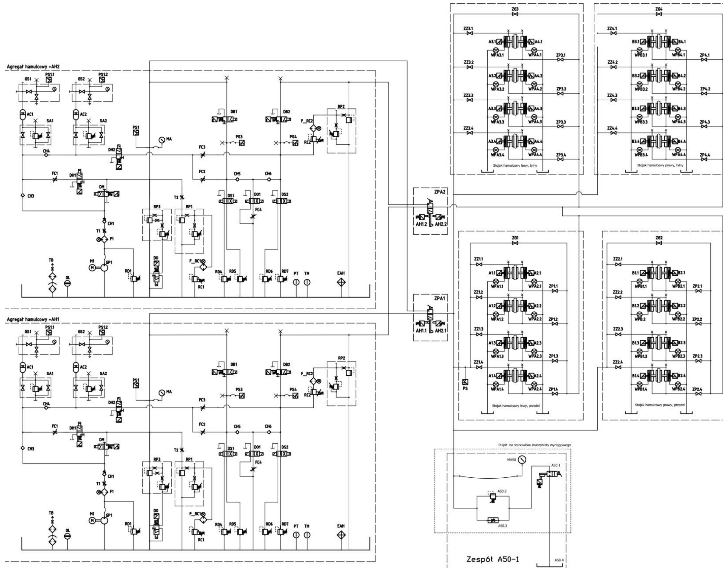
Schemat połączenia agregatów z silownikami wraz z przełącznicą agregatów ZPA1, ZPA2 oraz zespołem awaryjnego zatrzymania maszyny wyciągowej A50-1
