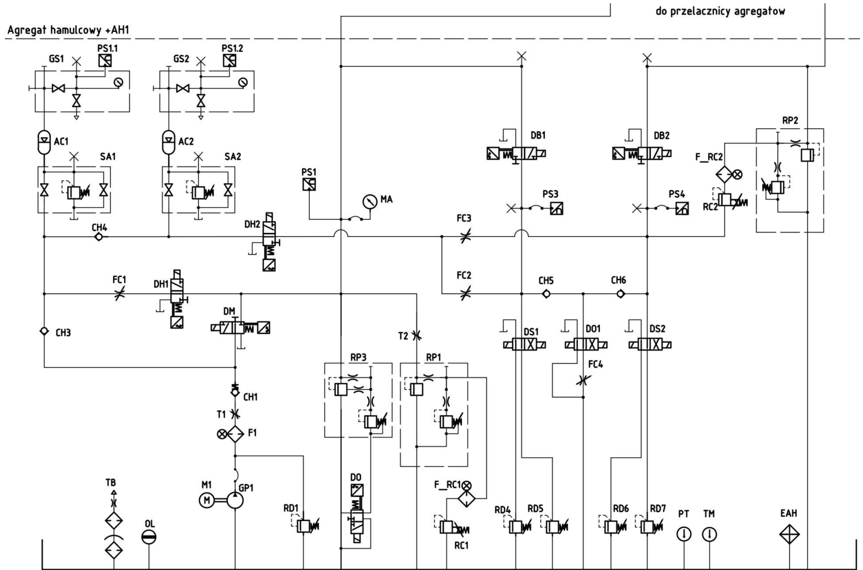
Schemat sterowania układu hamulcowego – agregatu AH1
