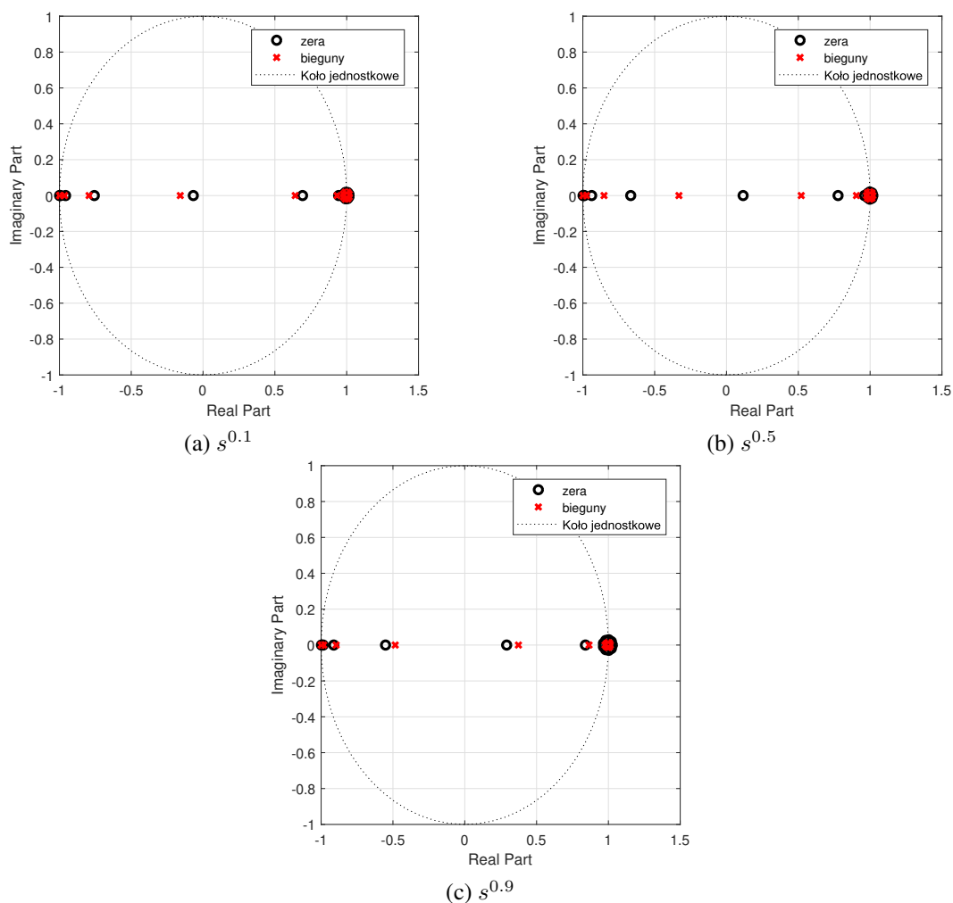
Rysunek 1: Rozkład zer i biegunów systemów dyskretnych dla aproksymacji czasowego Oustaloup rzędu 15
