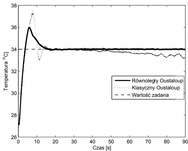
Rysunek 6: Porównanie wydajności kontrolerów dla stałej wartości wymuszenia
