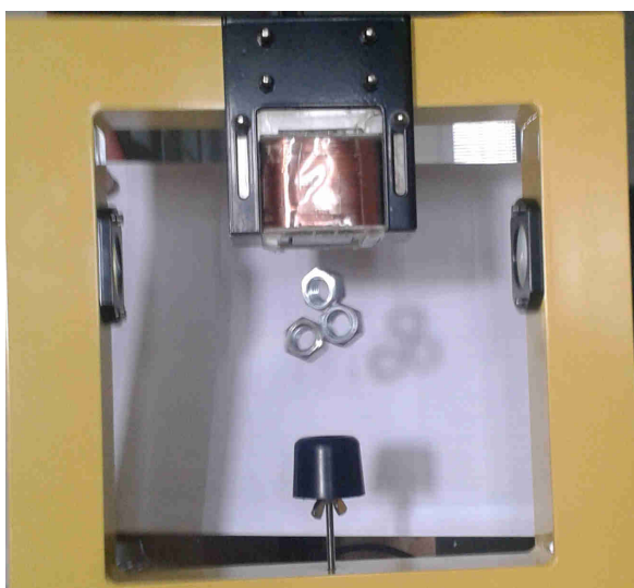
Rysunek 14: Nakrętki lewitujące w systemie z regulatorem PI^{\lambda}D
